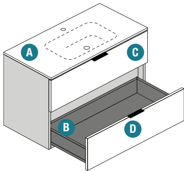
Maniglia FILO FILO Handle Poignée FILO FILO Griff
