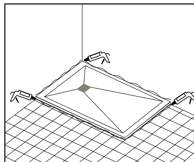
SCELLAGE / ABDICHTUNG
